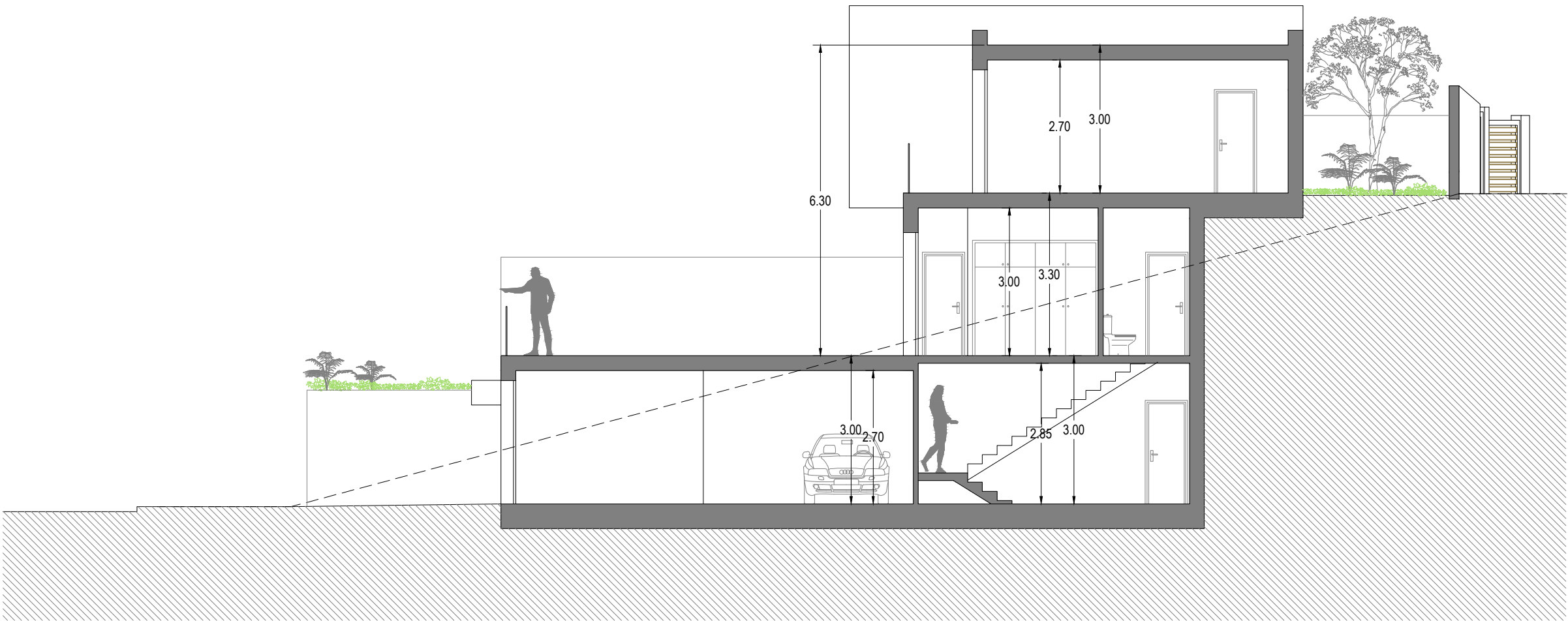
SECCION KK'
