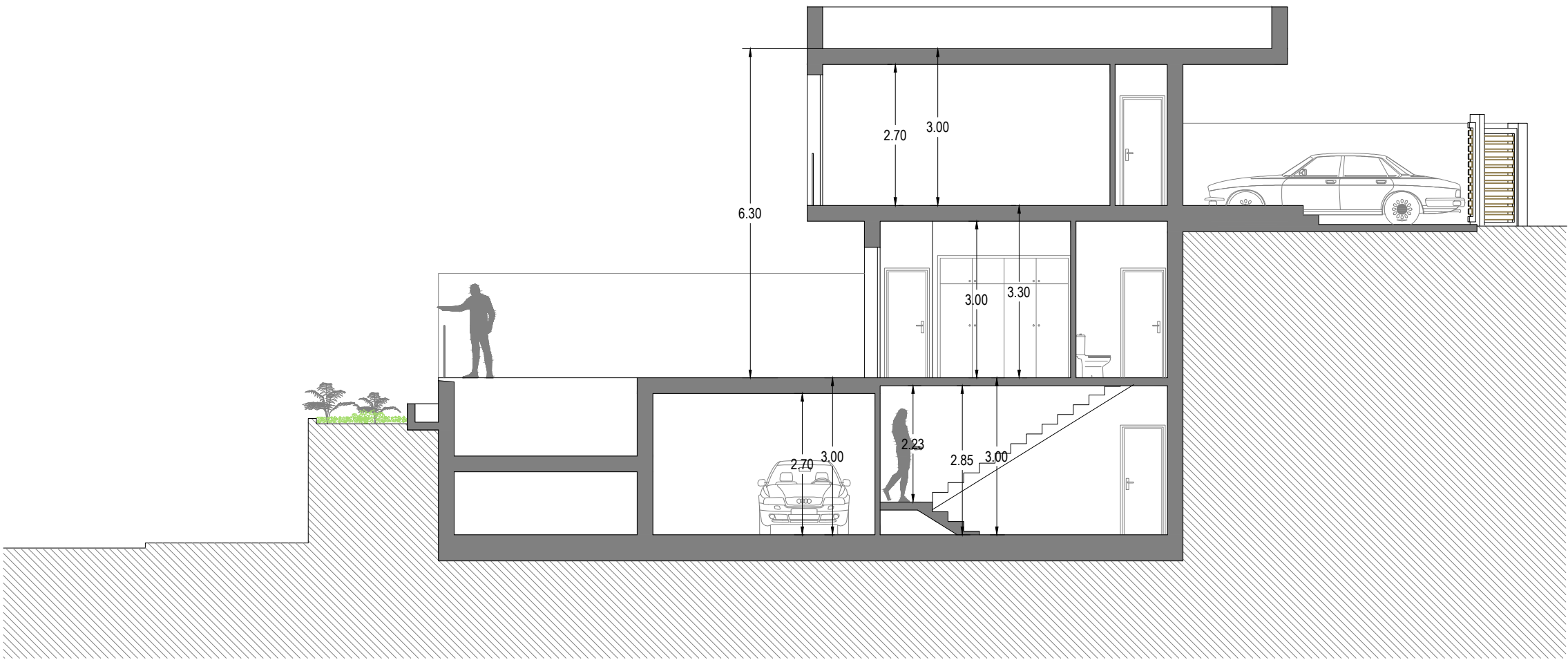
SECCION LL'
