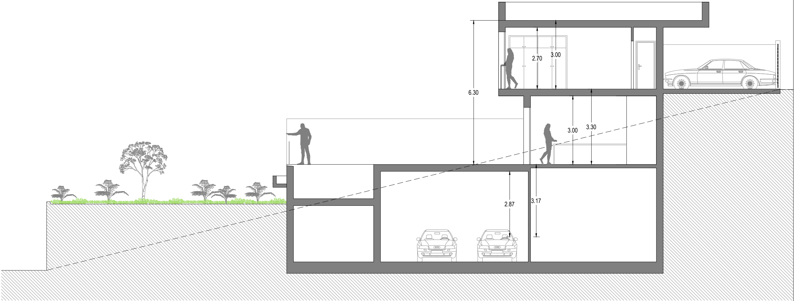
SECCION HH'
