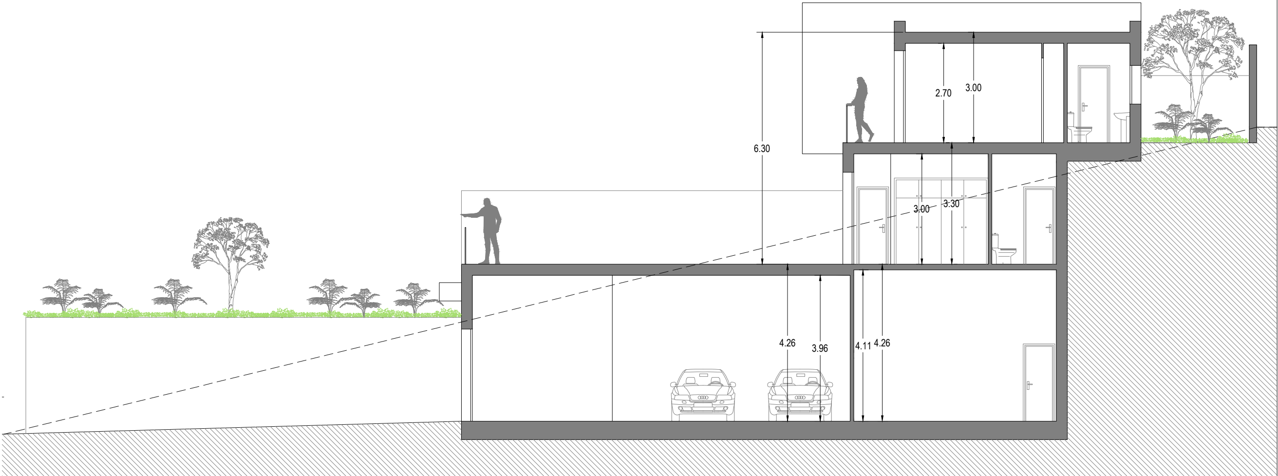
SECCION GG'
