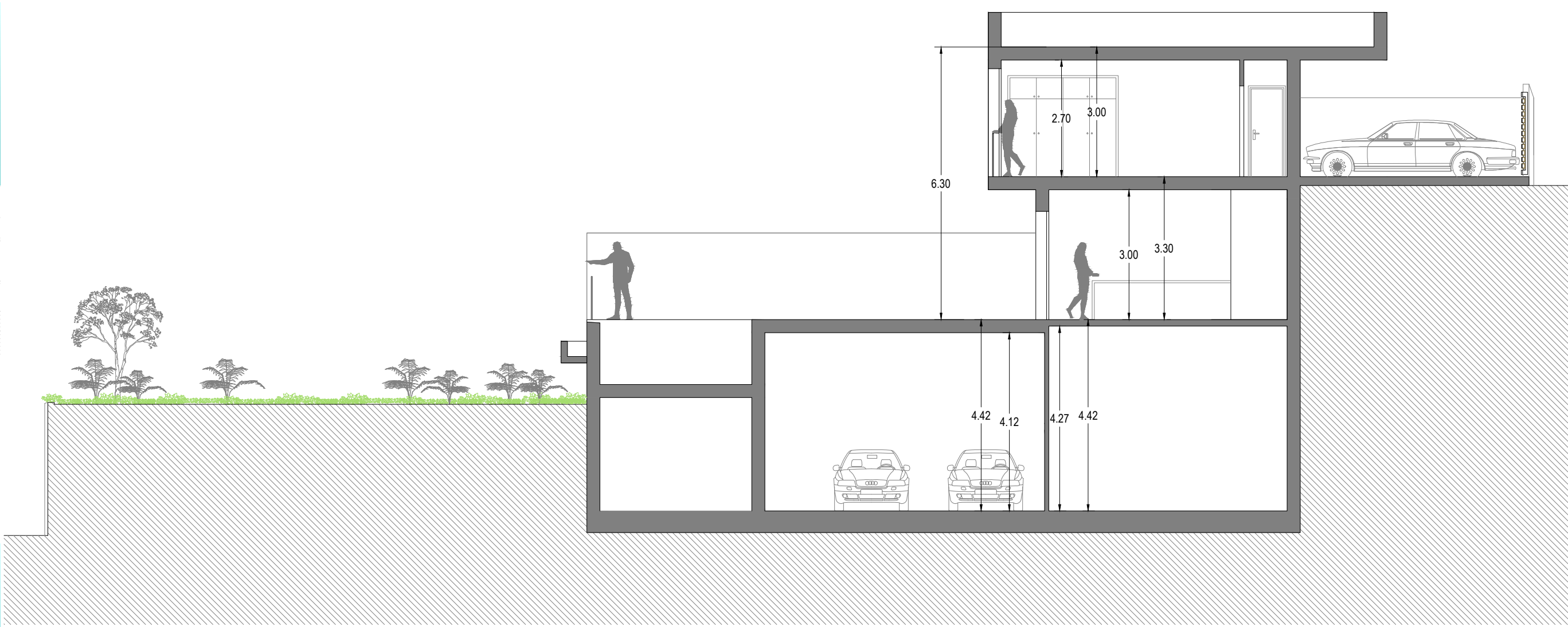
SECCION FF'
