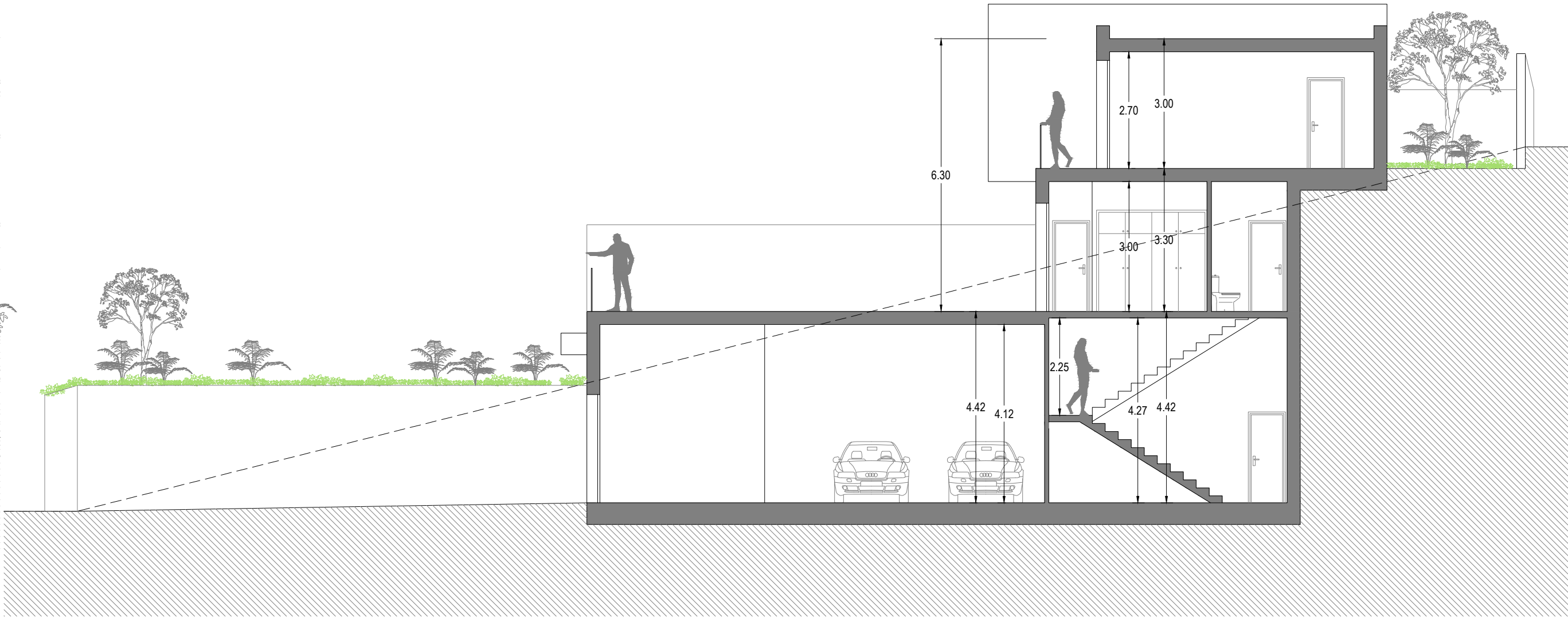
SECCION EE'
