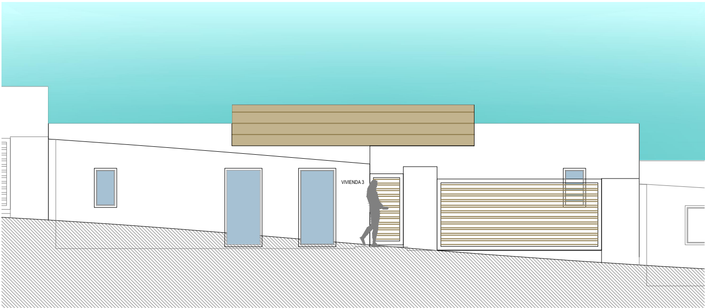
ALZADO OESTE
