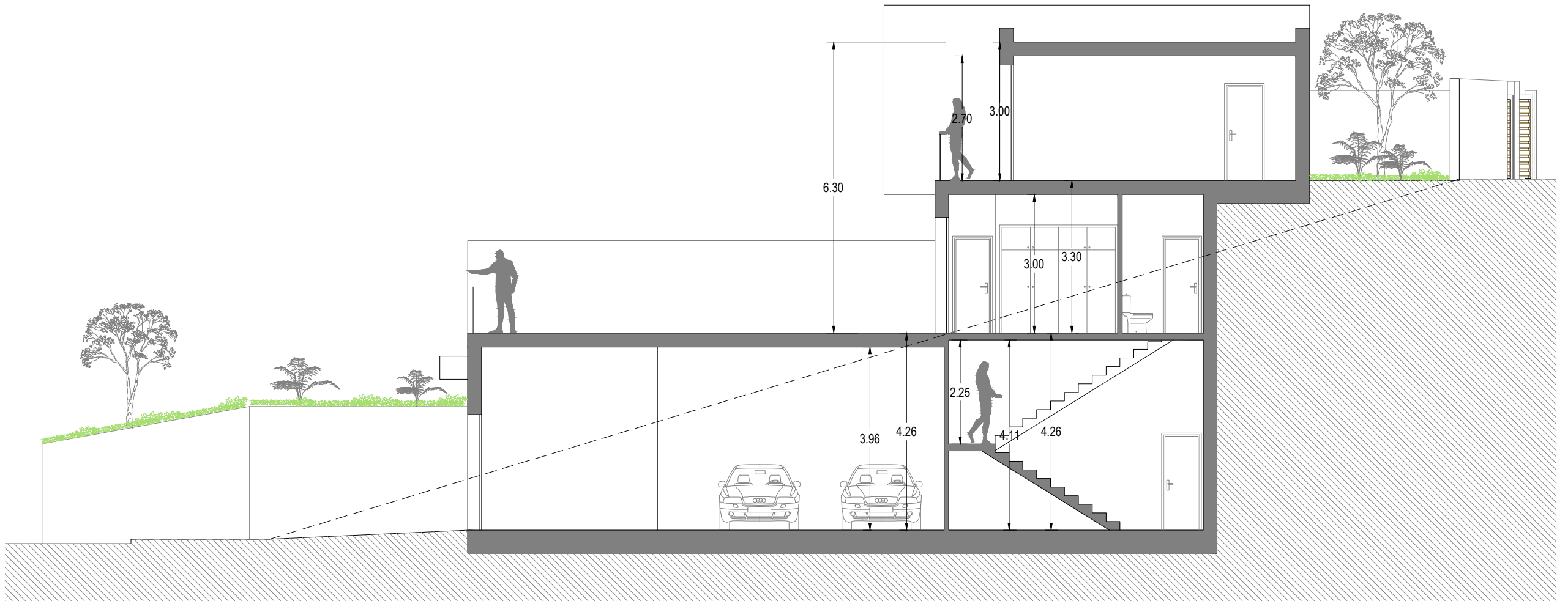
SECCION CC'
