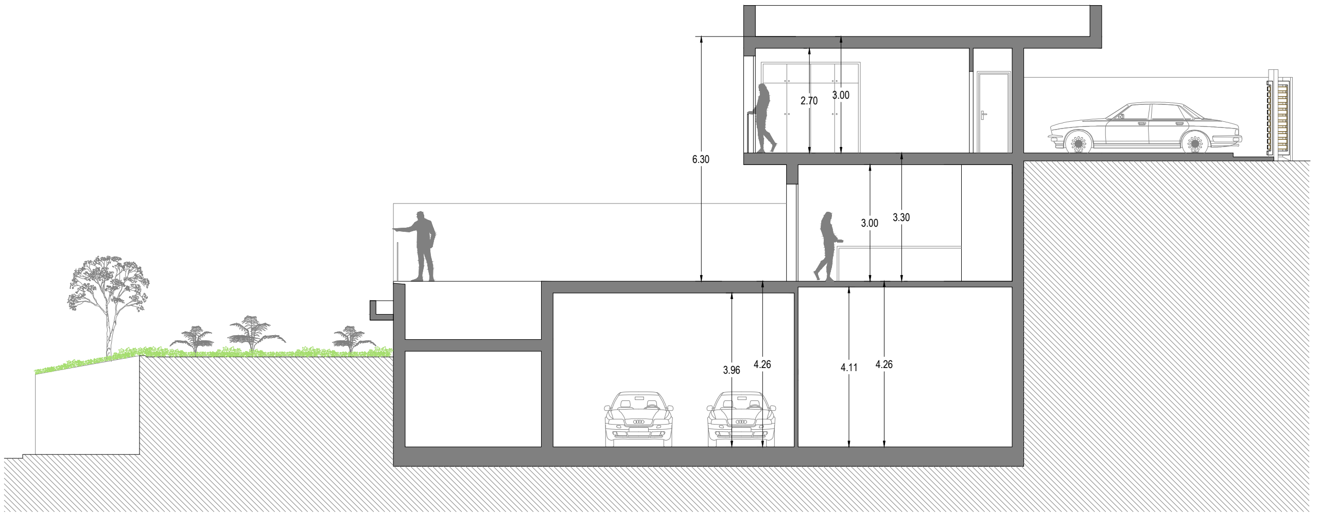
SECCION DD'
