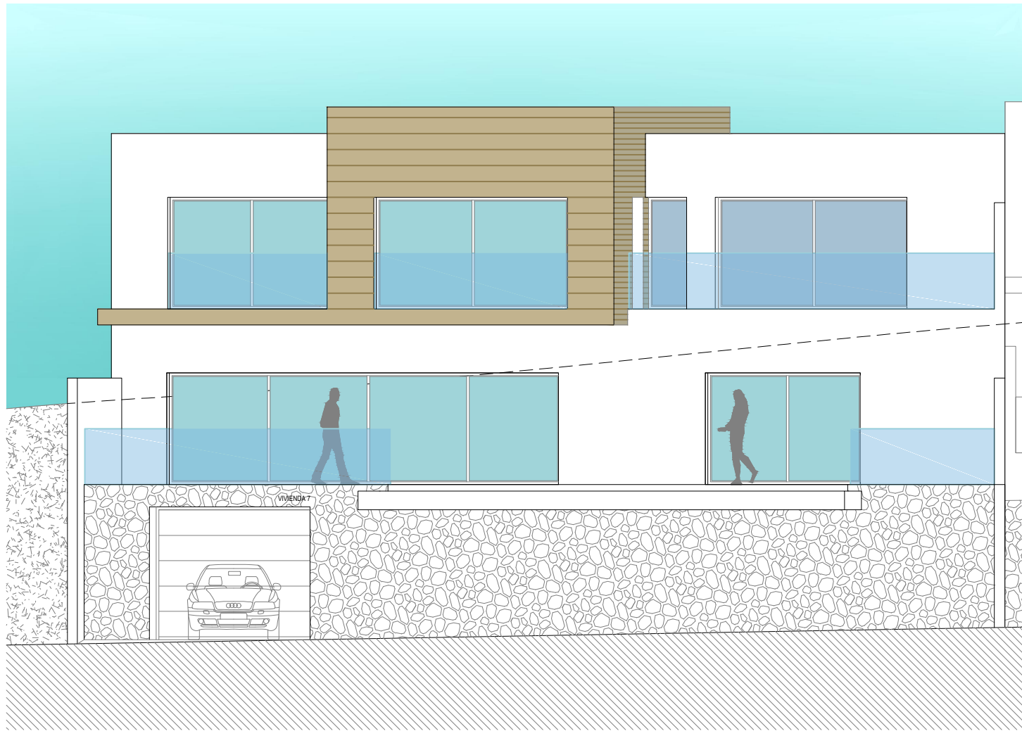
ALZADO ESTE
