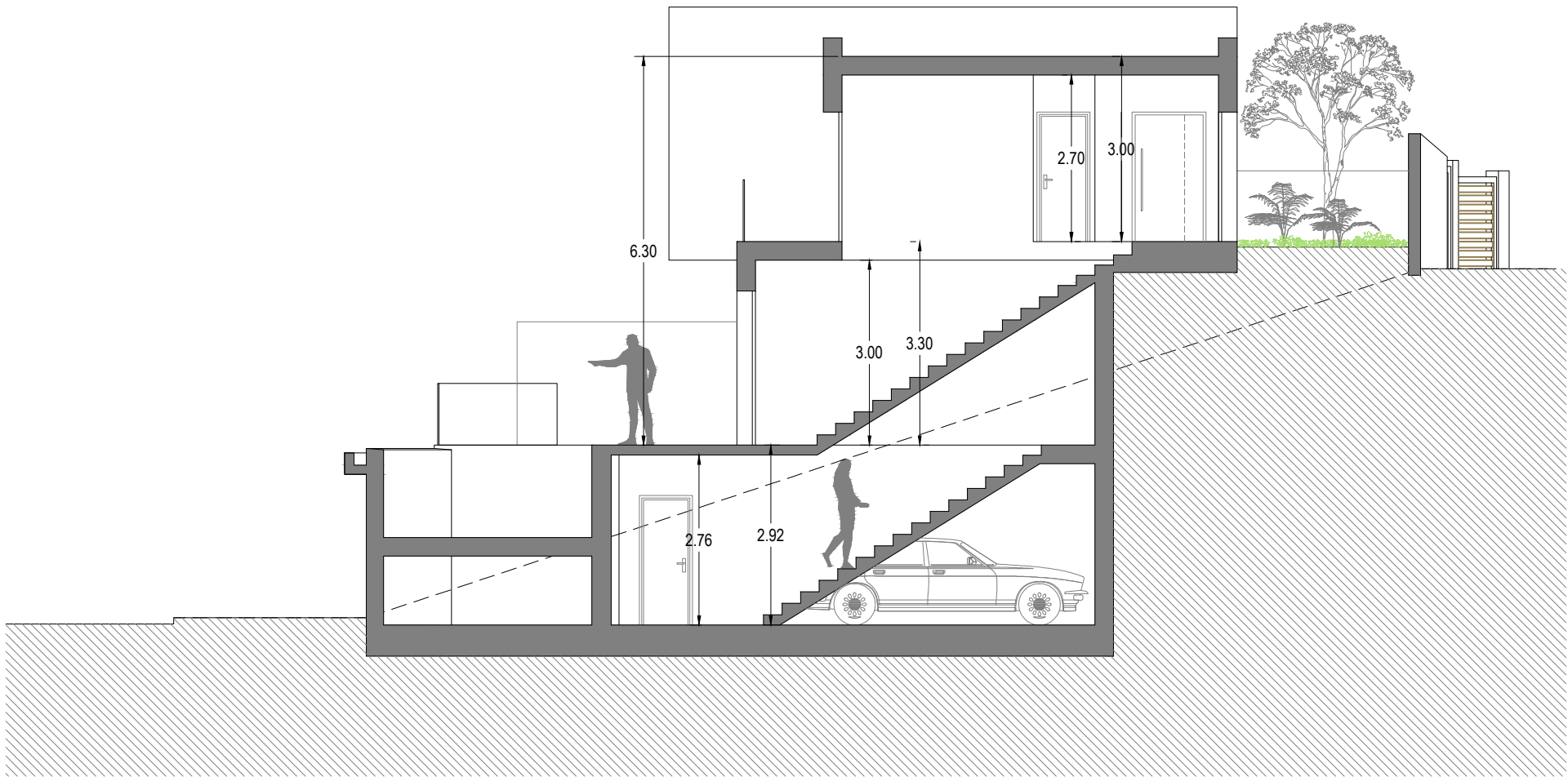
SECCION MM'
