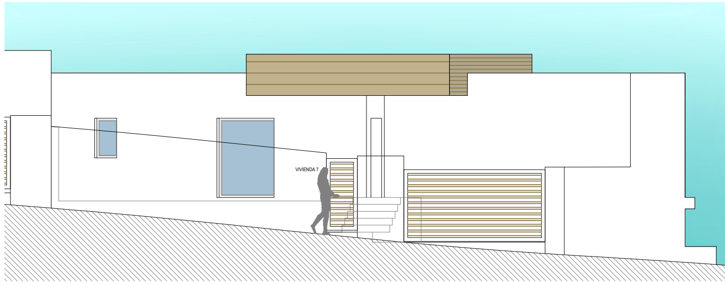
ALZADO OESTE
