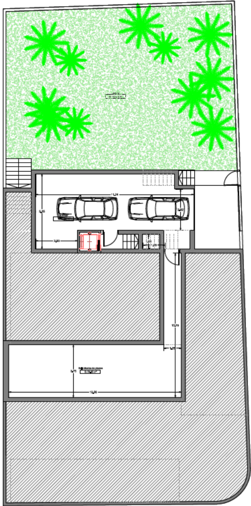
PLANTA GARAJE
