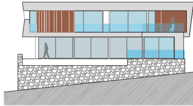
ALZADO SUR
