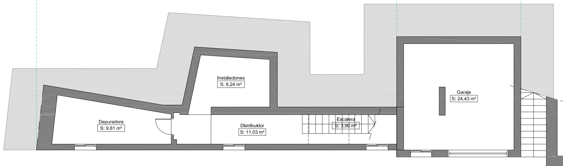
ENTREPLANTA
