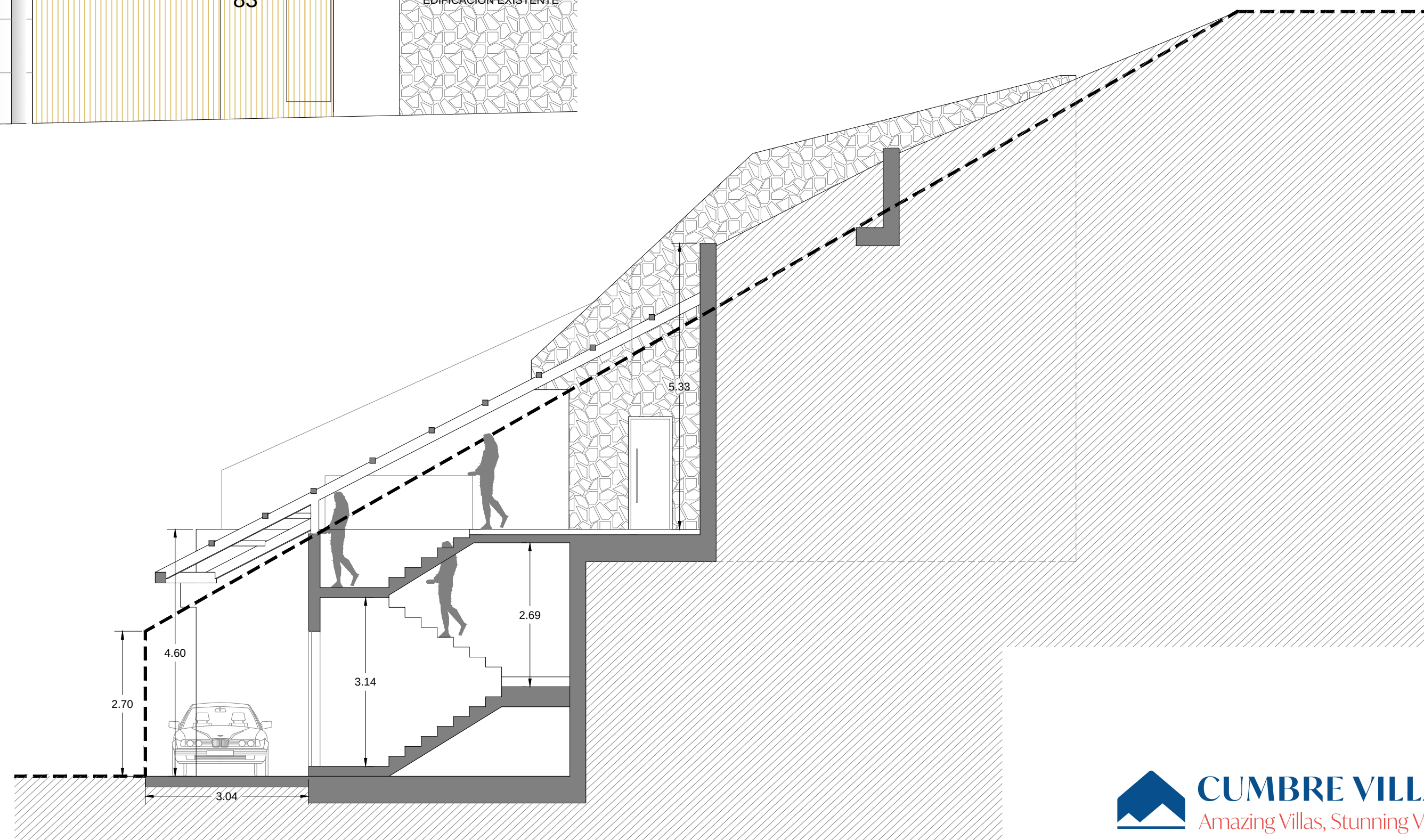
SECCION AA'
