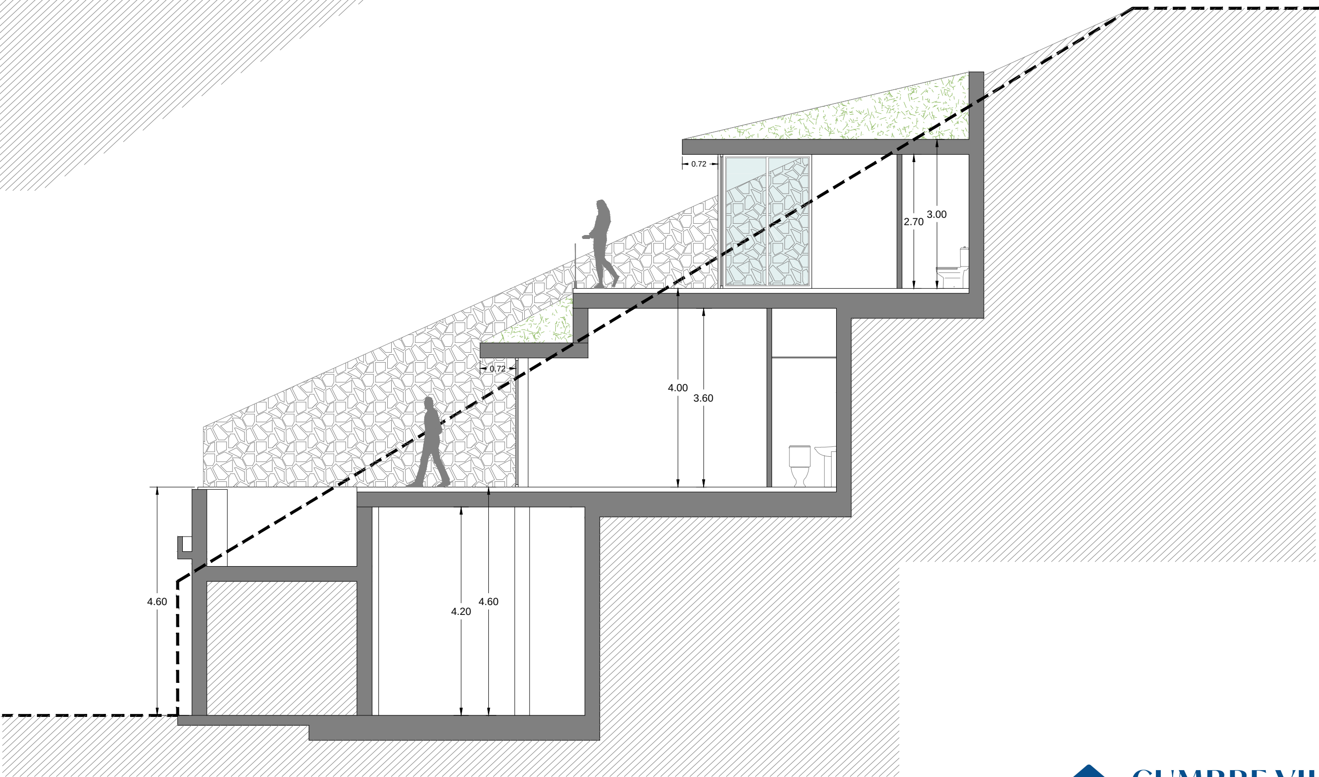
SECCION BB'
