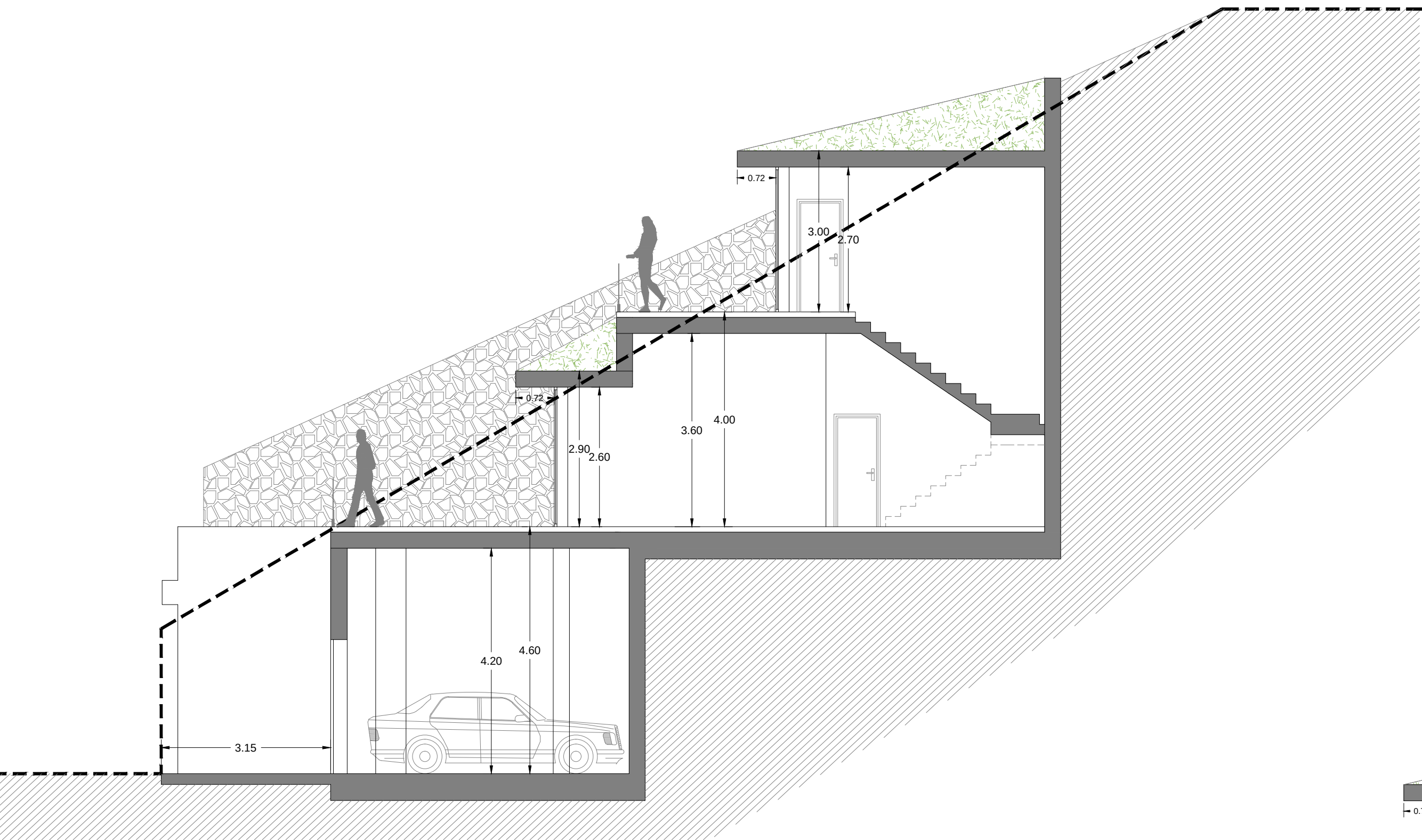
SECCION CC'
